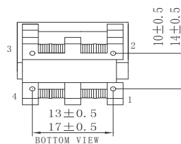
卧式 (H4)
